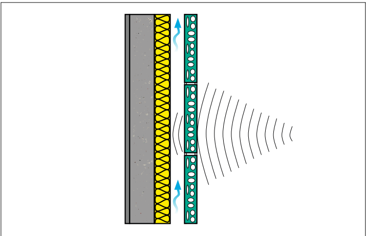
Insonorisation. Schalldämmung
