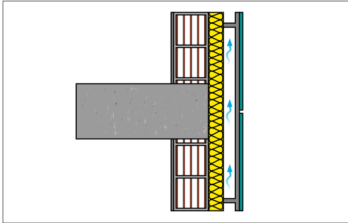
Ventilazione. Aeration
