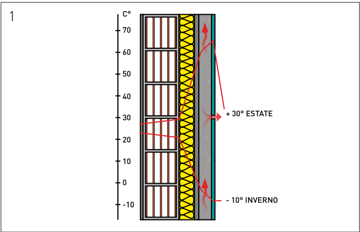
Tendance de la température à l’intérieur du mur pendant les saisons d’hiver et d’été (1); effet de la protection contre le rayonnement solaire direct pendant la saison estivale et schématisation de l’activation de la ventilation en (2) Temperaturtrend innerhalb der Wand während der Winter- und Sommersaison (1); Wirkung der Abschirmung vor Sonneneinstrahlung direkt während der Sommersaison und Schema der Aktivierung der Belüftung in (2)
