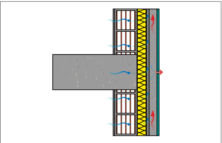
Transfert de l’excès de vapeur d’eau de l’intérieur du bâtiment dans l’environnement extérieur. Übertragung von überschüssigem Wasserdampf aus dem Inneren des Gebäudes in die Außenumgebung.
